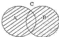
Hình 2. A \cup B
