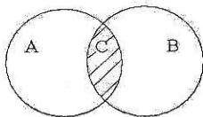
Hình 1. A \cap B
